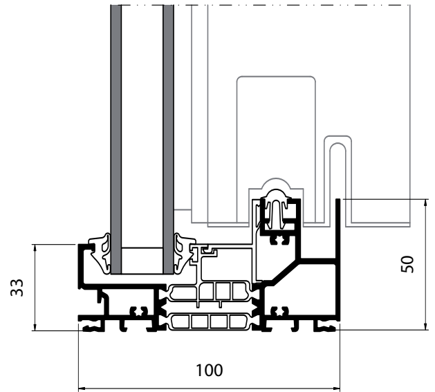
Coupe verticale
