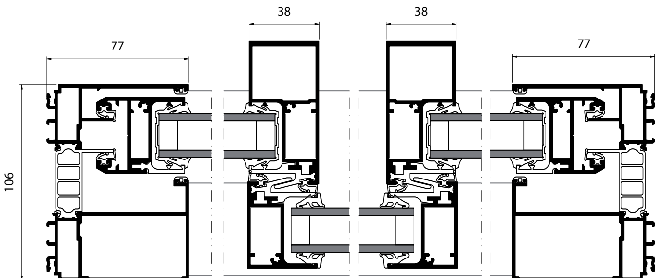
Coupe horizontale
