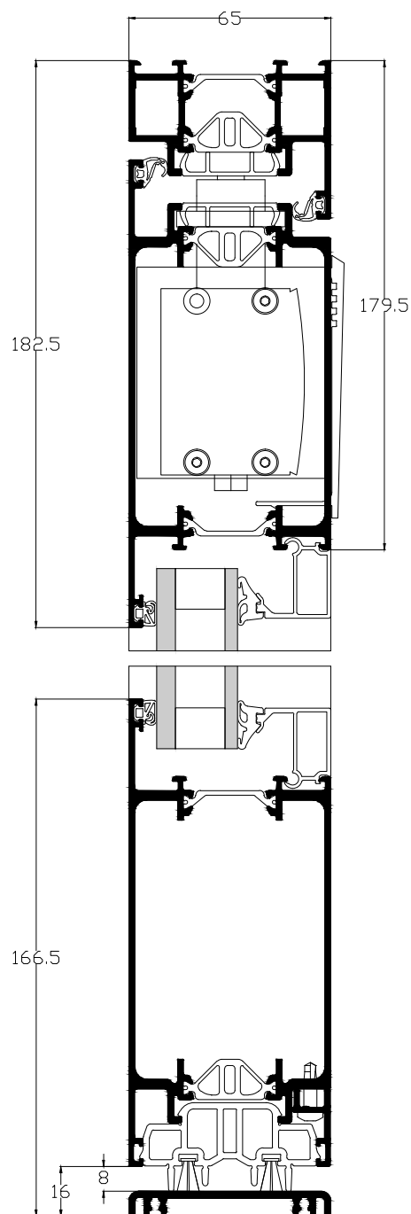
Coupe verticale 1C-C'
