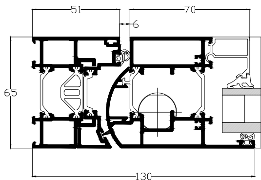
Coupe horizontale 1 B-B'
