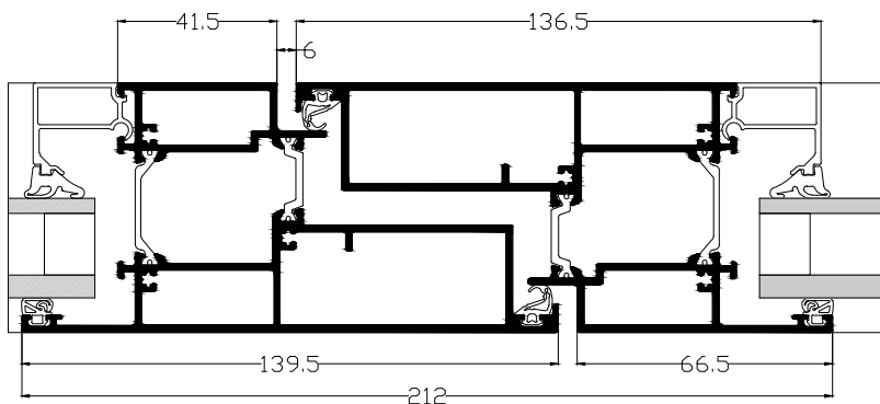
Coupe horizontale 1 A
