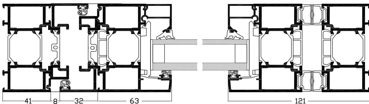
Coupe horizontale 1 B B'
