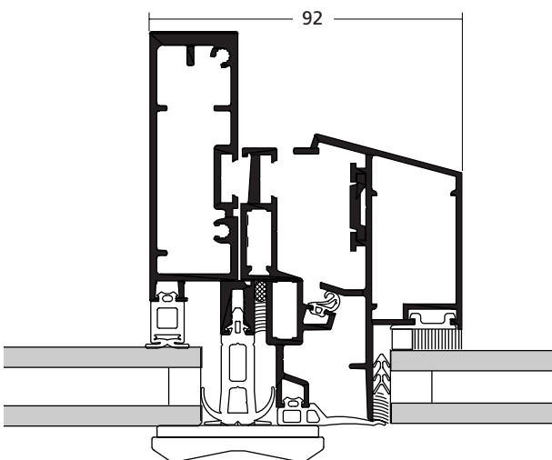
Coupe horizontale 1 B
