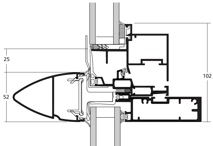
Coupe verticale «ouvrant accès pompier»
