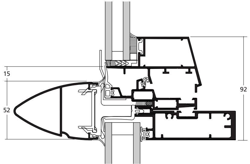
Coupe verticale oscillo-battant 1 A
