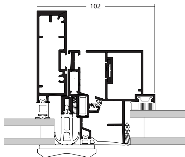
Coupe horizontale «ouvrant accès pompier»
