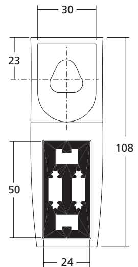
Coupe horizontale 1-A
